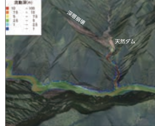
天然ダム決壊シミュレーション
