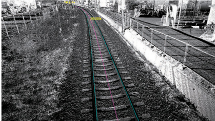
RaiLisIによるレーザ点群と設備自動抽出
