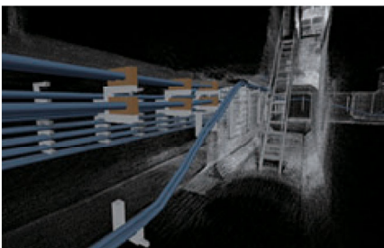
変電所地下設備の3次元モデル化
